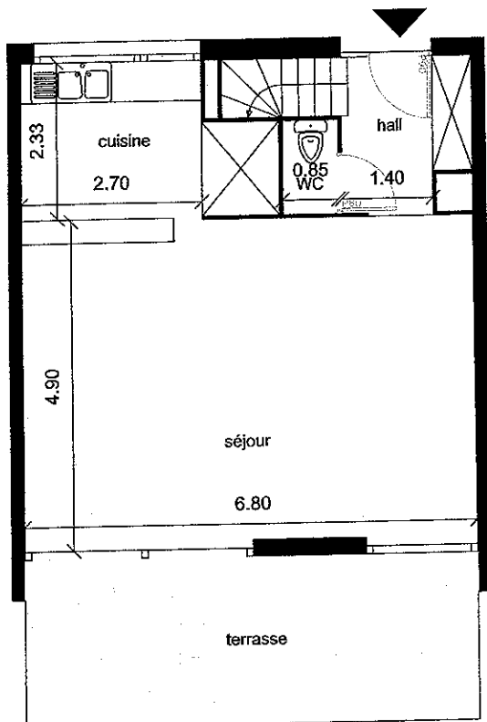
plan au rez-de-chaussée
