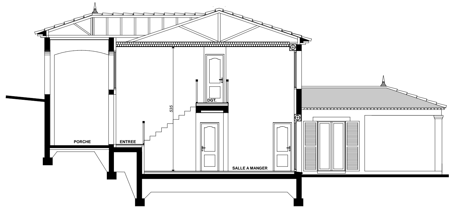
COUPE ENTREE - SALLE A MANGER
