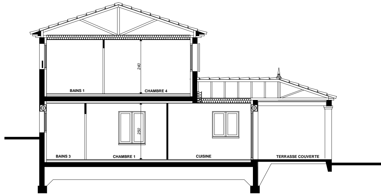
COUPE BAINS 3 - CUISINE
