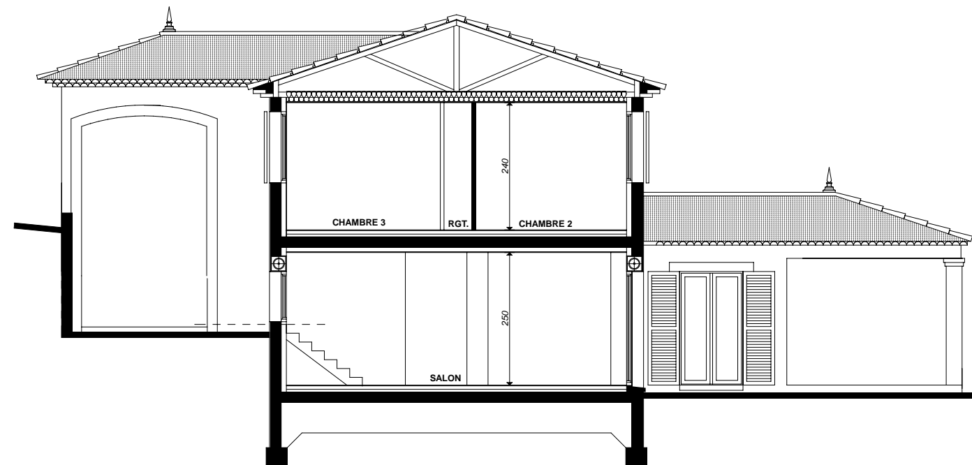
COUPE SALON
